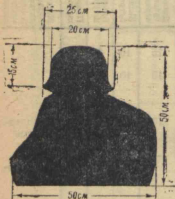
№ 12. Грудная (уменьшена в 10 раз)
