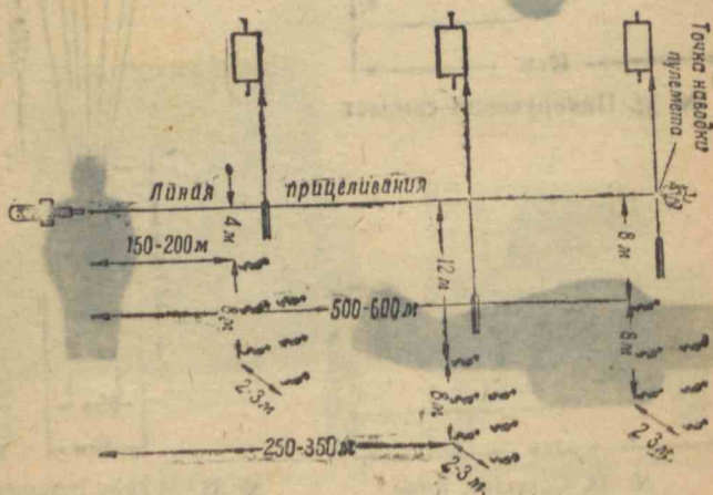
Рис. 2. Установка целей для 4-го упражнения учебных стрельбы в составе подразделений
