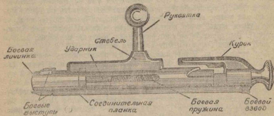
Рис. 2. Затвор в собранном виде
