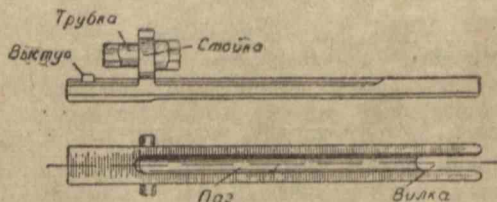
Рис. 10. Соединительная планка
