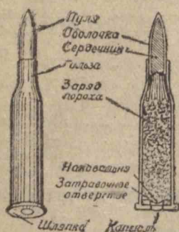
Рис. 3. Боевой патрон, общий вид и разрез
