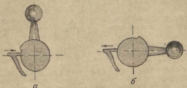
Рис. 14. Рукоятка затвора повернута влево. Лопасть отсечки-отражателя попала в глубокую часть скошенного паза стебля затвора (а). Рукоятка повернута вправо. Лопасть отсечки-отражателя попала в менее глубокую часть скошенного паза стебля затвора и отжалась влево (б)
