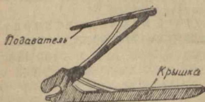
Рис. 12. Крышка магазинной коробки с подающим механизмом
