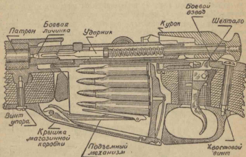
Рис. 5. Разрез винтовки. Положение патронов и частей в заряженной винтовке
