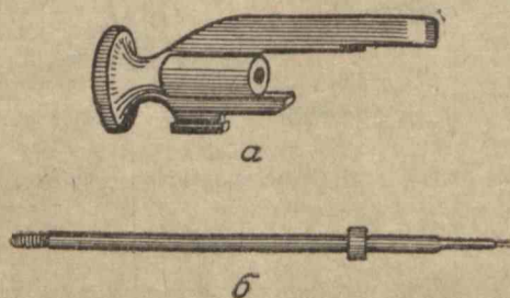
Рис. 6. а — курок, б — ударник
